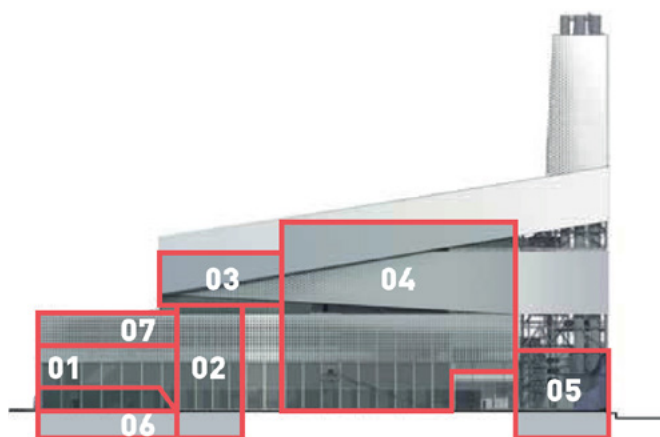
01 - Quai de déchargement des ordures ménagères. 02 - Fosse de réception des ordures ménagères. 03 - Garage. 04 - Four - chaudière et traitement des fumées. 05 - Groupe turboalternateur de production d'électricité. 06 - Parc de stationnement. 07 - Locaux des équipes de l'exploitant.
